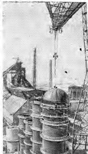
Один за другим вступают в строй действующих объекты Западно-Сибирского металлургического завода (Кемеровская область). За короткий срок здесь построены первая доменная печь, две коксовые батареи. НА СНИМКЕ: общий вид строительства второй доменной печи.
