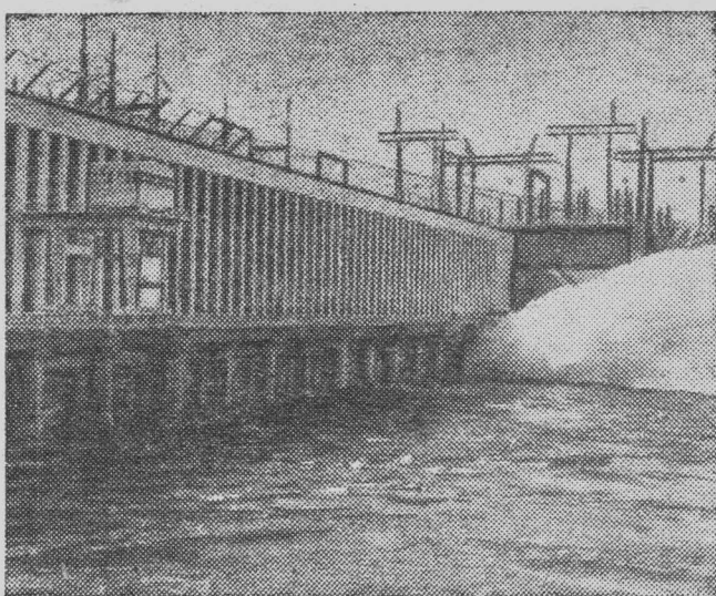
ОАР. В январе 1971 года завершено строительство крупнейшего в Африке Асуанского гидроэнергетического комплекса на Ниле, сооруженного при экономическом и техническом содействии Советского Союза.
