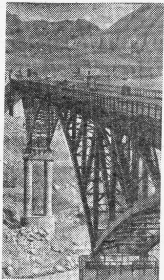
Алтайский край. В Онгудайском районе на Чуйском тракте закончен монтаж автогужового моста через реку Катунь. Мост собран из специальных конструкций и представляет собой новинку в отечественном мостостроении.
