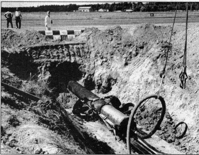
Машина для проколов земляного полотна работает на реконструкции взлетно-посадочной полосы
